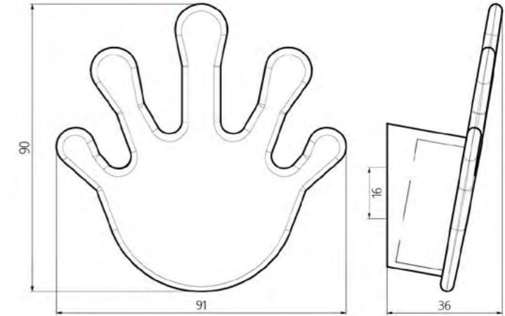
3.5x30
