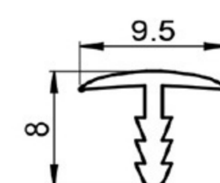
EDGE PROFILE
